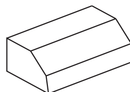
Cordón tope de rueda a: 35 h: 20 l: 60
