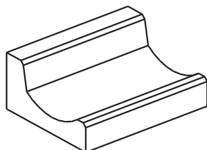
Cordón cuneta a: 46 h: 25 l: 60
