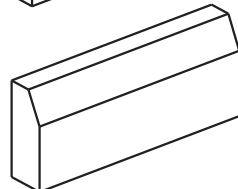
Cordón de contención a: 10 h: 25 l: 70
