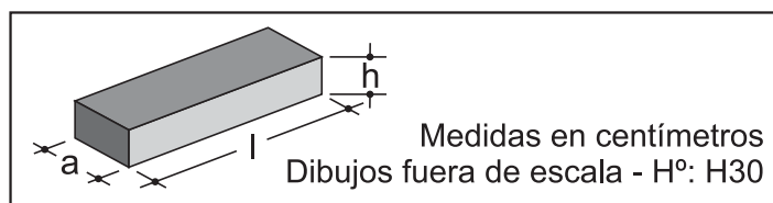
Cordón YPF a: 30 h: 10 l: 50
