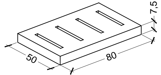
TAPA CANALETA 50 x 80
