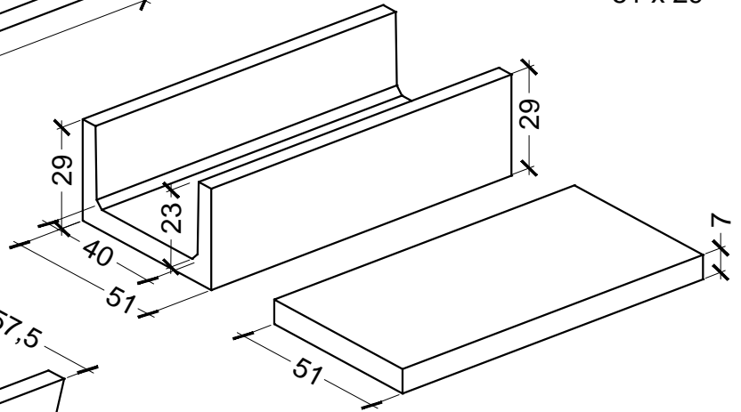
CANALETA SIN RAJA H°A° 51 x 29
