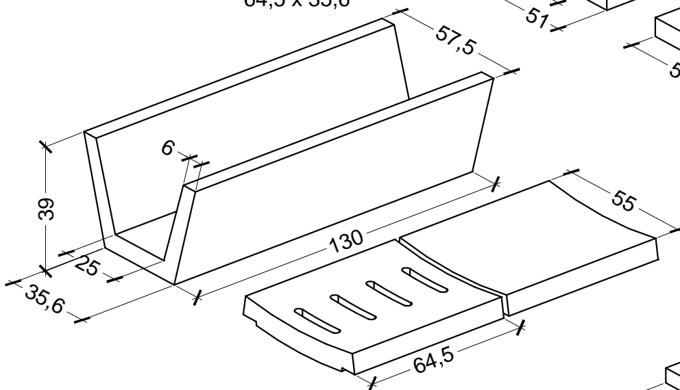
CANAL PREMOLDEADO H°A° 64,5 x 35,6
