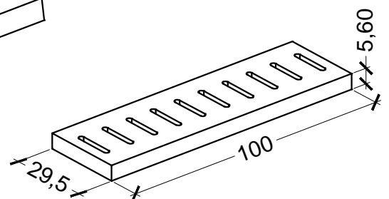
TAPA CANALETA 100 x 29,5
